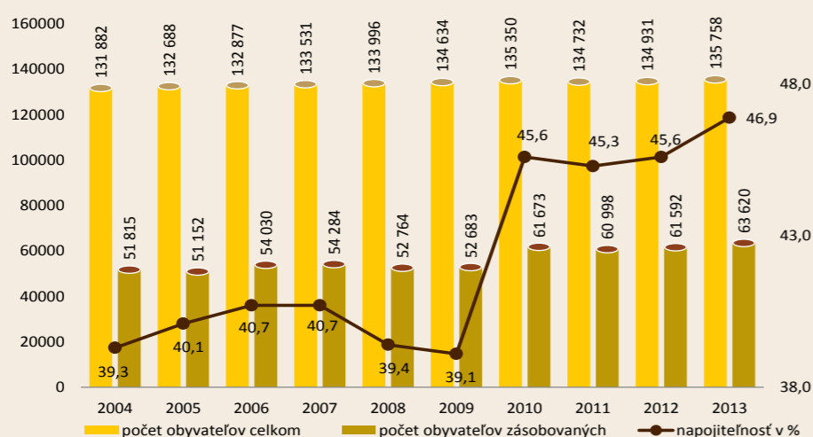
Obyvatelia celkom, obyvatelia nehnuteľností napojení na verejnú kanalizáciu, % napojiteľnosti
