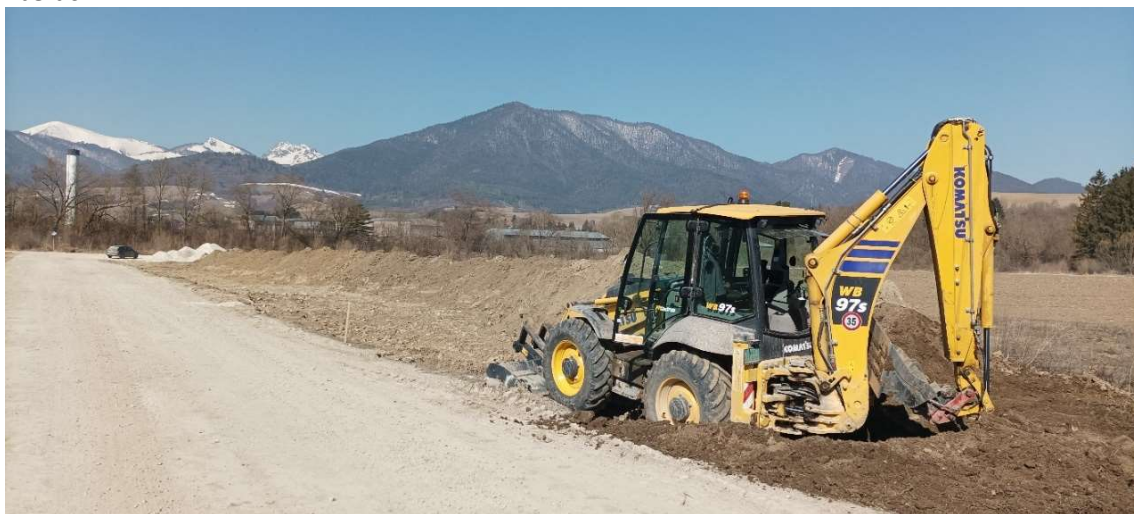
Obr.4: Výkopové práce na SS.05 Žaškov – Oravská Poruba, kanalizačný zberač
