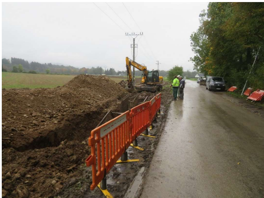
Obr. 9: Výkop ryhy pre uloženie kanalizačného potrubia PP DN400, stoka A (SS.07)
